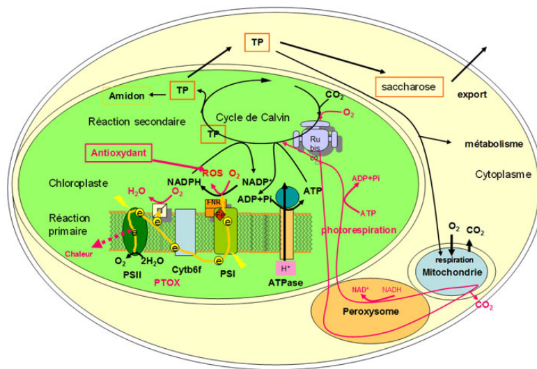
Figure 4. Représentation schématique d'une cellule chlorophyllienne montrant quelques aspects de la coopération entre chloroplaste, cytoplasme (avec les mitochondries et les peroxysomes), et les principaux complexes protéiques impliqués dans la photosynthèse. L'absorption de la lumière et le transport électronique dans la réaction primaire de la photosynthèse, lié à la membrane des thylacoïdes, sont montrés en jaune. Cette réaction inclut les complexes protéiques PSII, Cytochrome b6/f, PSI et ATPase. Les flèches noires montrent l'utilisation de l'énergie pour l'assimilation du CO 2 dans la réaction secondaire et pour la synthèse de sucres ainsi que leurs utilisations dans la cellule. Il y a aussi des voies alternatives d'utilisation de l'énergie absorbée (montrées en rouge), dont le fonctionnement peut protéger la photosynthèse : l'émission de l'énergie en excès sous forme de chaleur, la réduction de l'oxygène en eau par la protéine PTOX, la formation des ROS par le PSI et leur détoxification par les antioxydants, enfin la voie de la photorespiration initiée par l'absorption d'oxygène par la Rubisco. Pour les détails voir le texte. [Source : Schéma © Peter Streb]. Abréviations ; AT(D)P : Adénosine tri(di)phosphate ; Cytochrome b6/f ; e : électron - le transport des électrons entre le PSII et le NADP + est indiqué ; Fe : Ferrédoxine ; FNR : Ferrédoxine-NADP-Réductase ; NADP(+H) : Nicotinamide adénine di-nucléotide phosphate (+ forme oxydé, H forme réduite) ; PSI PSII : photosystème I et II ; PTOX : oxydase terminale plastidiale ; Rubisco : ribulose-bis-phosphate carboxylase oxygénase (complexe enzymatique qui catalyse la fixation du CO 2 ) ; SDP : sucrose-di-phosphate (substrat pour la Rubisco) ; TP : triose phosphate (premier sucre phosphorylé apparaissant après l'assimilation du CO 2 ).
